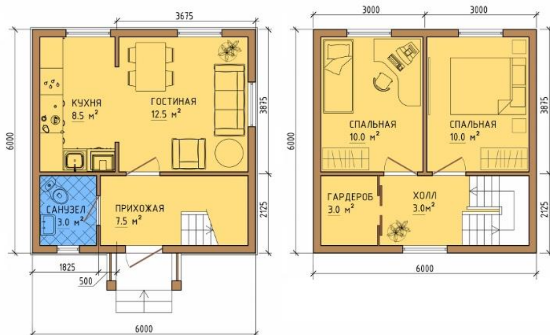
ПЛАНЫ ЭТАЖЕЙ
